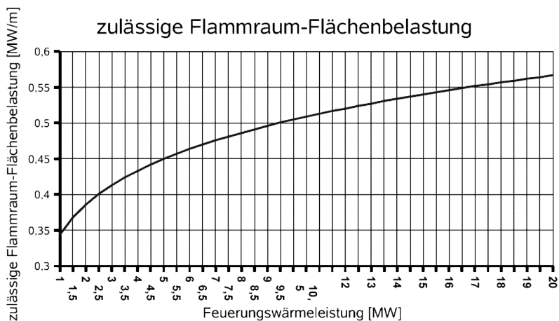
Bild 8: zulässige Flammraum-Flächenbelastung
