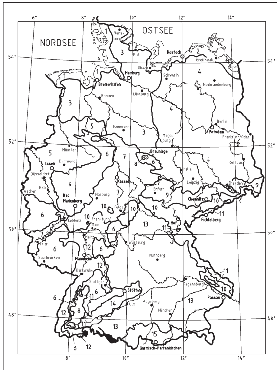
Klimazonen der DIN 4710:2003-01*)
