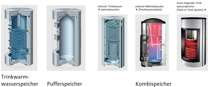
Abb. 3: den Ökodesign-Anforderungen unterliegende Warmwasserspeicher (EU-Verordnung Nr. 814/2013)
