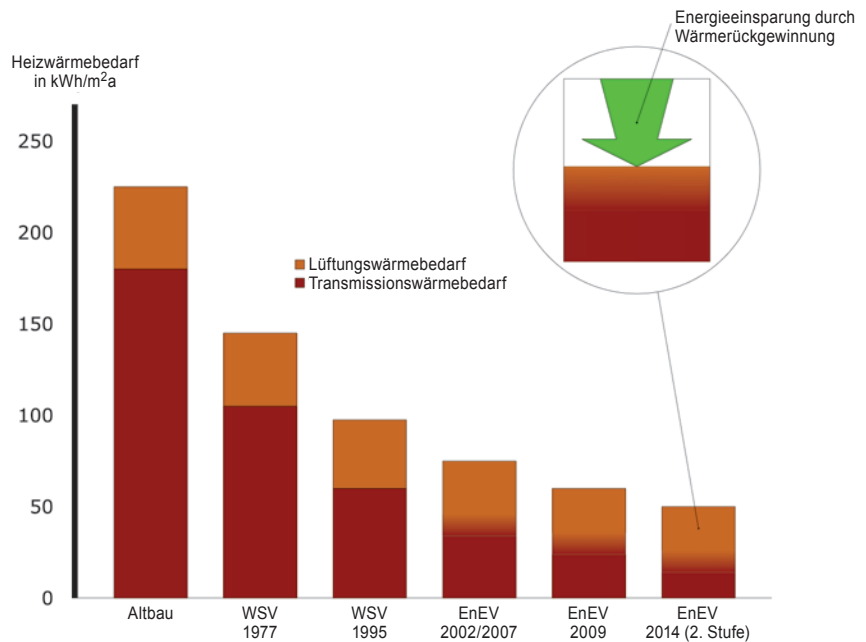
Bild 3: Relativer Anteil der Lüftung am Gesamtwärmebedarf
