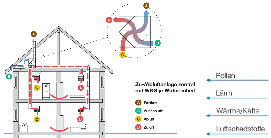
Bild 1 zeigt das Prinzip einer zentralen Lüftungsanlage mit Wärmerückgewinnung und die äußeren Einflüsse auf das Raumklima, die wirksam reduziert werden.
