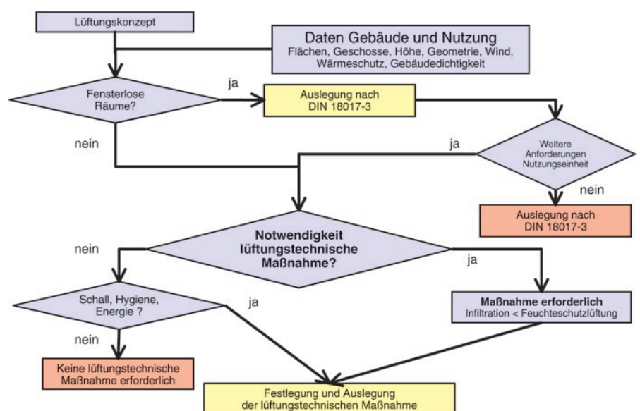
Bild 6: Vorgehensweise bei der Überprüfung der Notwendigkeit lüftungstechnischer Maßnahmen
