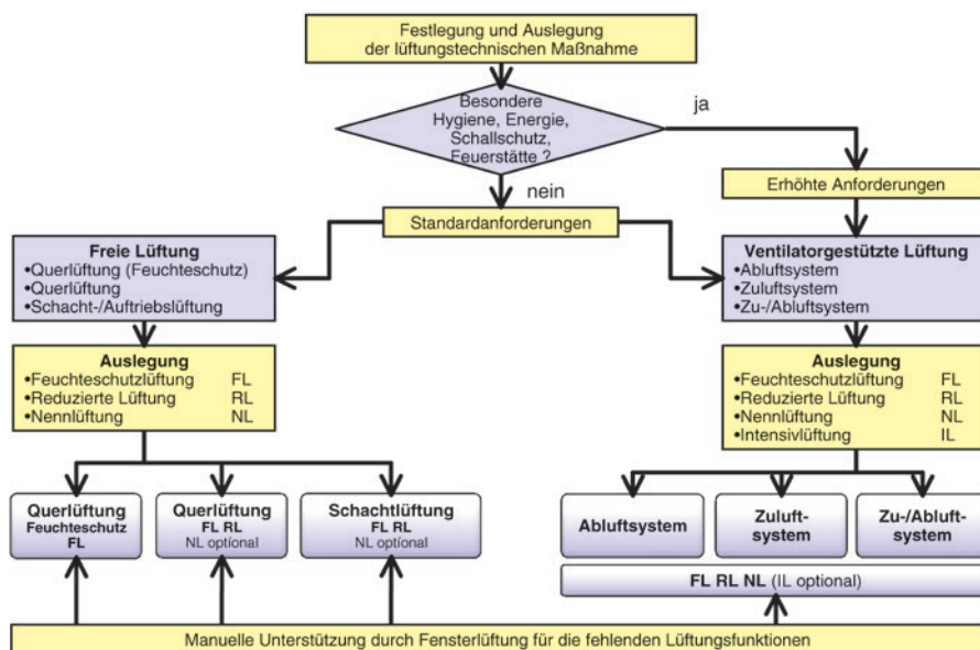
Bild 7: Varianten von Lüftungsanlagen
