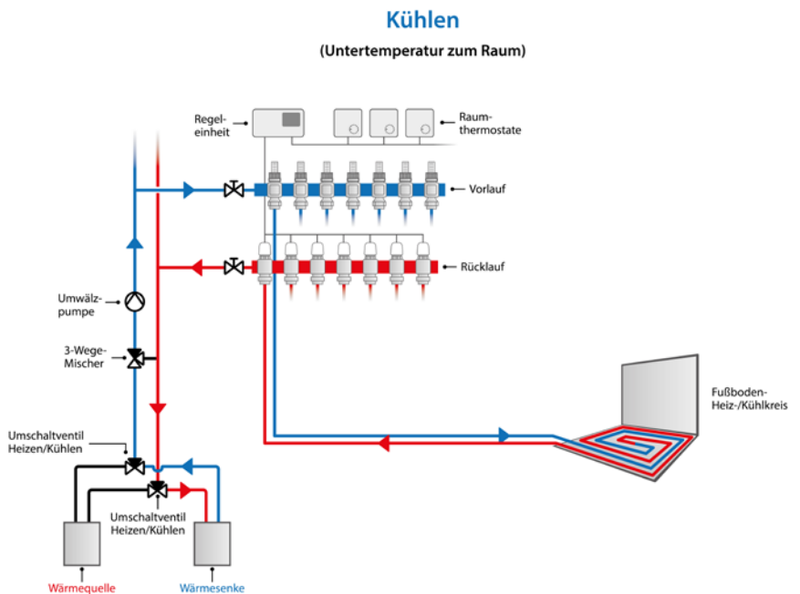
Abbildung 12: Typisches Anlagenschema für eine Fußbodenkühlung
