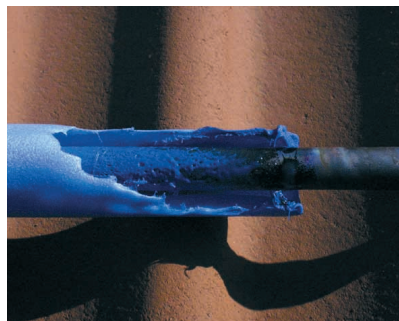
Bild 1: Aus der Heizungstechnik übliche Wärmedämmung ist für Solaranlagen nicht geeignet
