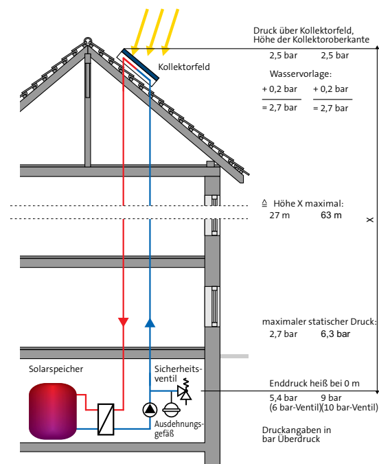
Bild 2: Druckverhältnisse im Kollektorkreis in Abhängigkeit der Gebäudehöhe beim Einsatz von Geräten unterschiedlicher Druckstufen im Keller
